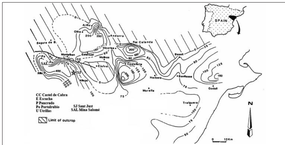
Figura 1. Localización del yacimiento y mapa de isopacas de la Fm. Escucha (tomado de Querol et al. , 1992)
