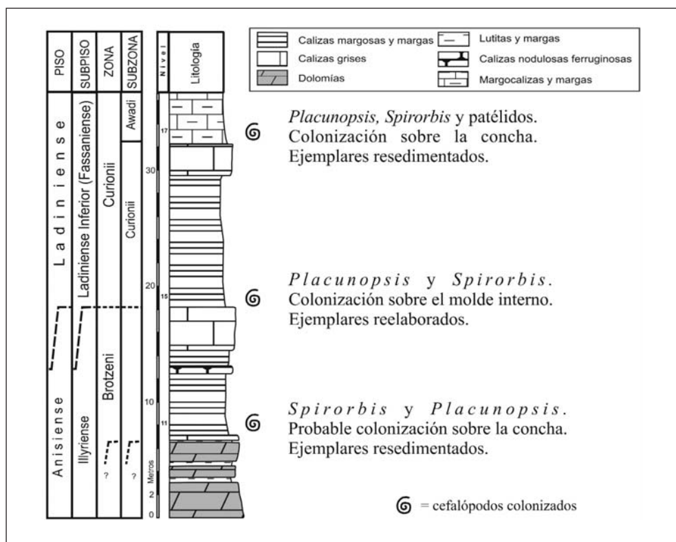
Figura 1. Intervalo estudiado de la sección de Calasparra (modificado de Pérez-Valera, J.A., 2005).
