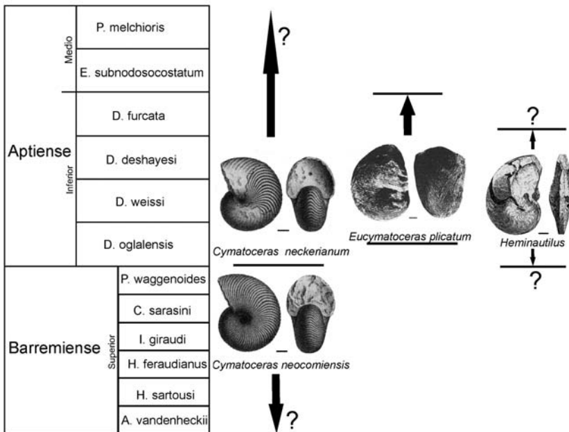
Figura 1. Propuesta sobre la distribución bioestratigráfica de los nautiloideos referida a las biozonas de ammonoideos de la biozonación mediterránea de Hoedemaeker et al. (2003).
